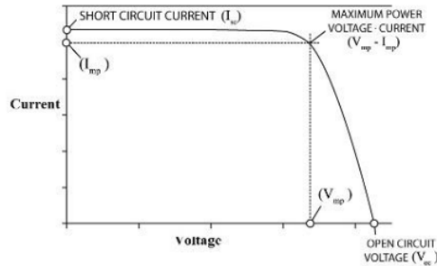
9 Gambar 12. Kurva I-V
