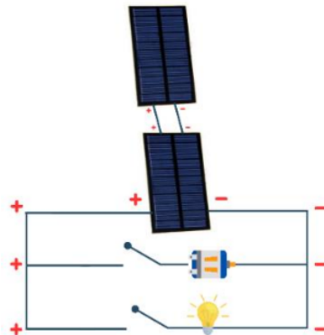
Gambar 5. Rangkaian listrik paralel pada alat peraga Mini Sopedric
